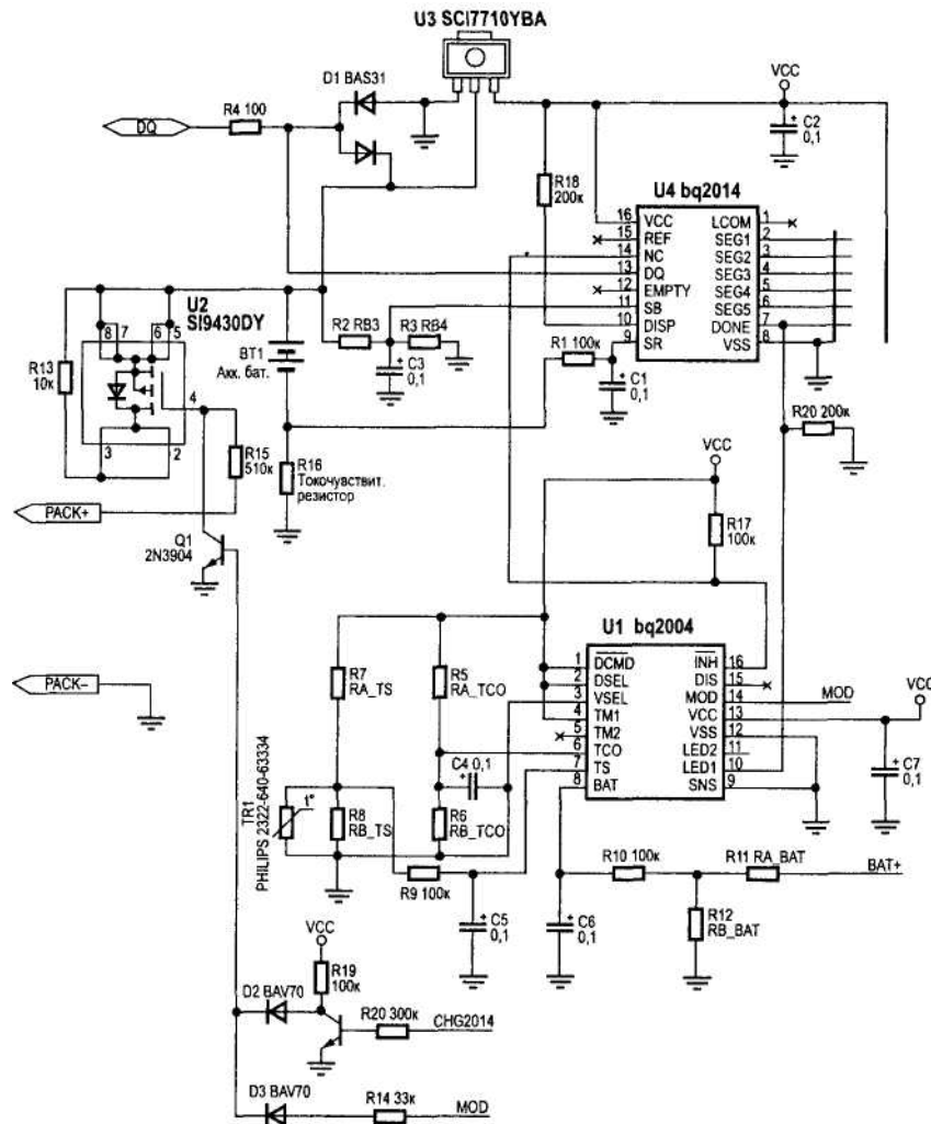
Рис. 8.7. Типовая схема зарядного устройства с устройством контроля емкости аккумуляторной батареи
