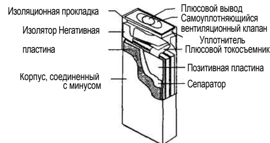
Рис. 2.5. Конструкция призматического аккумулятора
