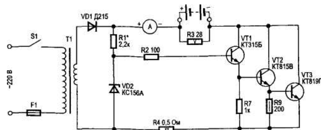
Рис. 8.16. Принципиальная схема устройства заряда асимметричным током
