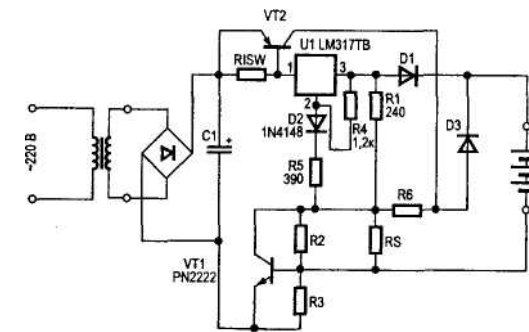
Рис. 8.17. Принципиальная схема устройства двухступенчатого заряда
