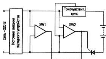
Рис. 3.8. Структурная схема зарядного устройства для двухступенчатого заряда
