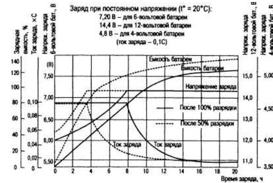
Рис. 3.6. Характеристики заряда при разряде батарей на 50 и 100 %
