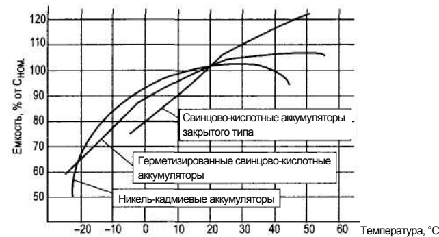
Рис. 7.9. Зависимость отдаваемой аккумуляторах емкости от температуры
