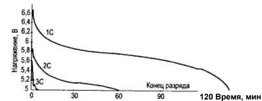
Рис. 7.3. Разрядные характеристики никель-металлгидридной батареи мобильного телефона
