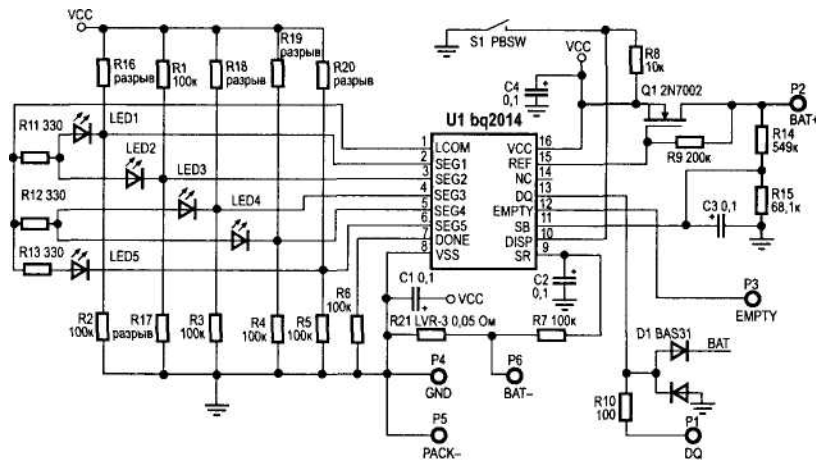
Рис. 8.8. Принципиальная схема устройства контроля емкости никель-металлгидридных батарей
