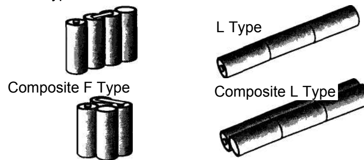
Рис. 2.7. Типы аккумуляторных батарей производства фирмы Panasonic
