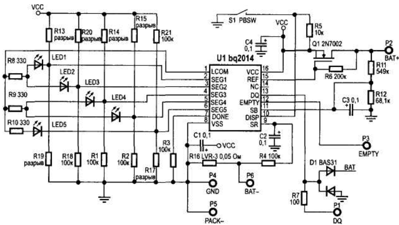
Рис. 8.9. Принципиальная схема устройства контроля емкости литий-ионных батарей
