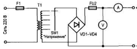
Рис. 8.12. Схема простого зарядного устройства свинцово-кислотных аккумуляторных батарей
