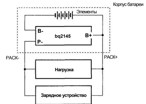
Рис. 8.10. Схема подключения модуля bq2145
