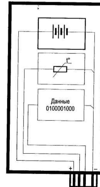
Рис. 6.1. Структурная схема Smart-батареи с 1-проводным интерфейсом 1-Wire®
