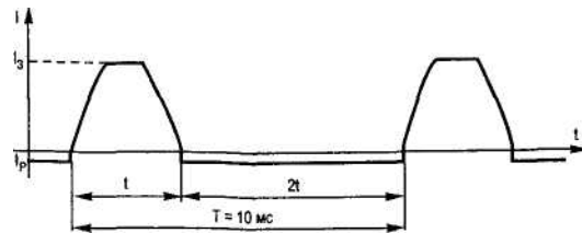
Рис. 8.15. Форма импульсов асимметричного тока заряда
