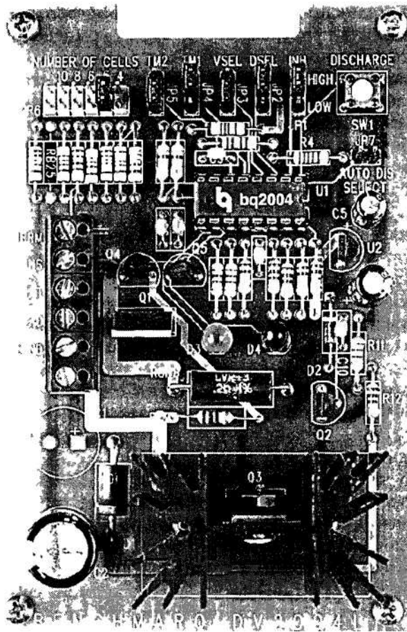
Фото 8 1 Плата из комплекта разработчика DV2004L1 для создания зарядных устройств на основе bq2004
