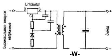
Рис. 9.6. Типовое включение LinkSwitch
