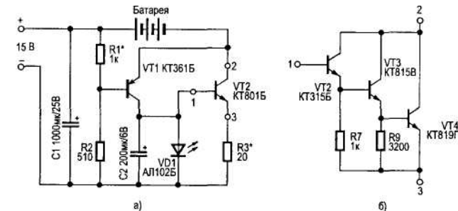
Рис. 8.14. Схема автоматического зарядного устройства для плавающего заряда свинцово-кислотных аккумуляторных батарей
