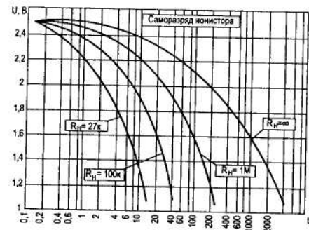
Рис. 5.3. Характеристики саморазряда ионистора
