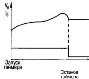
Рис. 2.15. Временная характеристика заряда с управлением по таймеру
