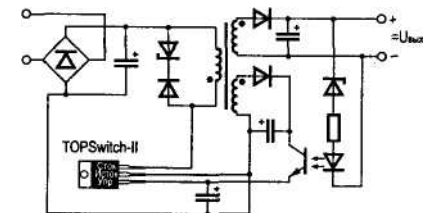
Рис. 9.2. Типовое включение TOPSwitch-II
