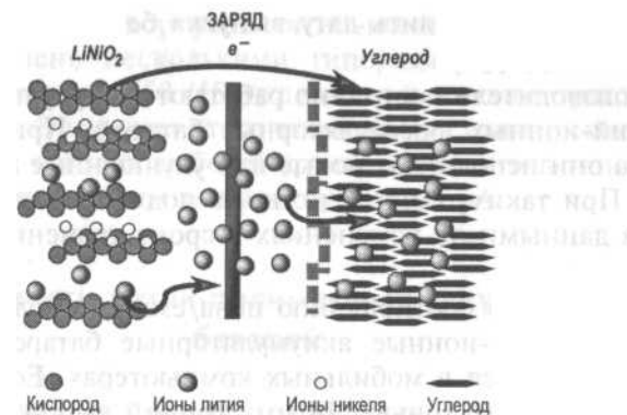
Рис. 4.2. Процесс заряда литий-ионного аккумулятора
