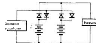
Рис. 7.8. Развязка ветвей аккумуляторной батареи при помощи диодов
