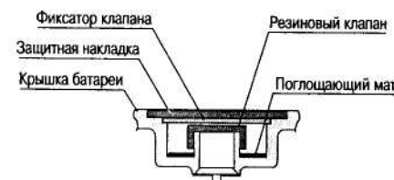
Рис. 3.5. Пример конструкции предохранительного клапана
