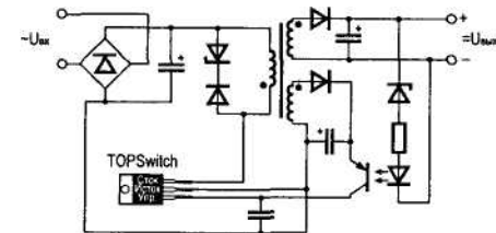
Рис. 9.1. Типовое включение TOPSwitch
