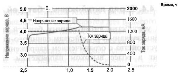
Рис. 4.6. График цикла заряда литий-ионного
