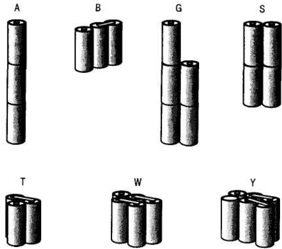
Рис. 2.9. Конфигурации аккумуляторных батарей GP и соответствующие им коды
