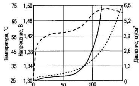
Рис. 2.22. Зарядные характеристики никель-кадмиевого аккумулятора
