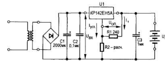
Рис. 8.13. Схема простого зарядного устройства на основе интегрального стабилизатора напряжения
