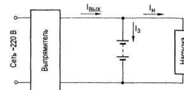
Рис. 3.11. Система с зарядкой батареи методом плавающего заряда
