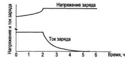
Рис. 3.7. Характеристики заряда при постоянных значениях напряжения и тока заряда
