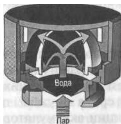
Рис. 3.14. Конструкция пробки с каталитическими насадками батарей Varta
