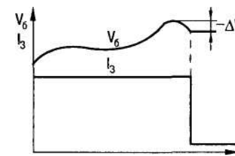
Рис. 2.18. Временная характеристика \Delta V -заряда Скоростной заряд током 0,5С ( t=10...40 С)
