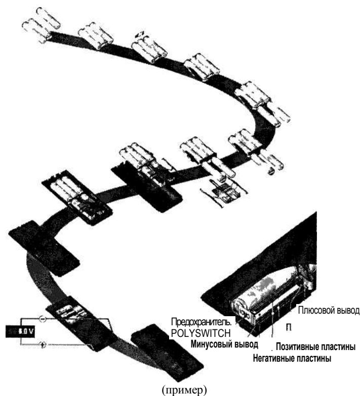
Рис. 2.6. Процесс сборки аккумуляторных батарей для мобильных телефонов
