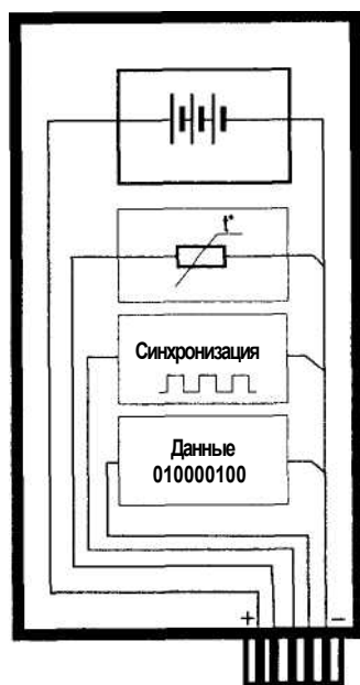
Рис. 6.2. Структурная схема Smart-батареи с шиной SMBus
