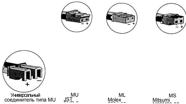
Рис. 2.10. Внешний вид соединителей для подключения батарей к печатным платам
